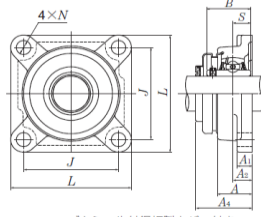
ゴムシール付鋼板製カバー付き
